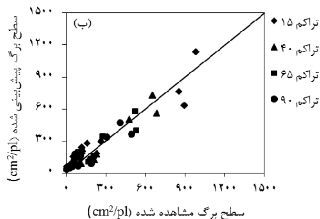
شکل ۱- رابطه بین سطح برگ و تعداد برگ در ساقه اصلی (الف) و رابطه بین سطح برگ مشاهده شده و سطح برگ پیش‌بینی شده (ب). O، مقادیر مشاهده شده و P، مقادیر پیش‌بینی شده در تراکم‌های ۱۵، ۴۰، ۶۵ و ۹۰ بوته در مترمربع
